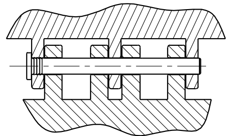
安装实例： 用于汽车的插销门把手
